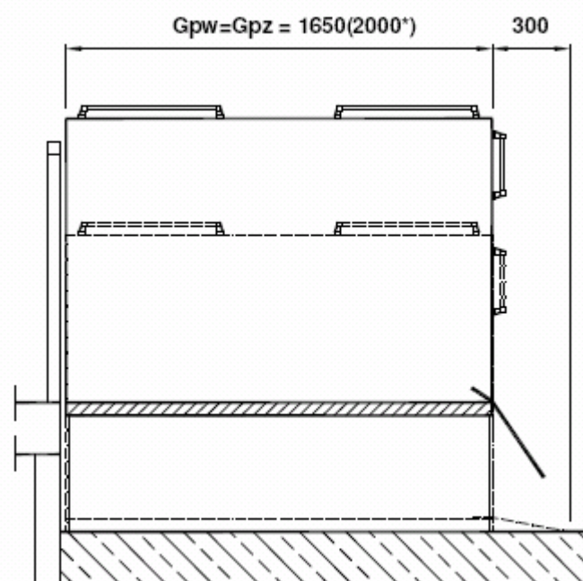
Rys. 1 Przekrój pionowy
